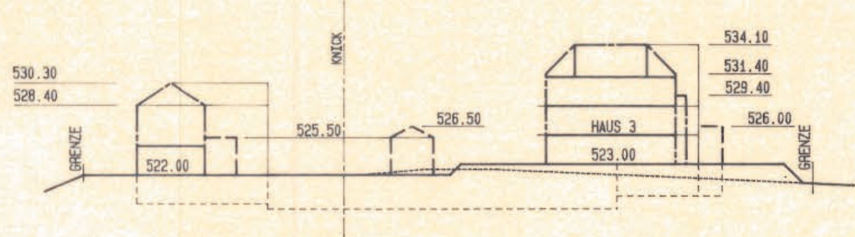
SCHNITT 02
