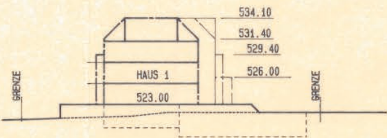
SCHNITT 04
