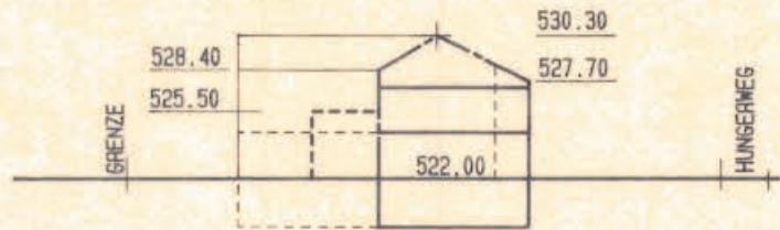
SCHNITT 01
