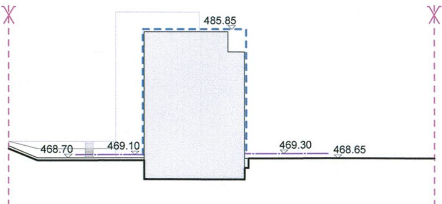
Schnitt A-A
