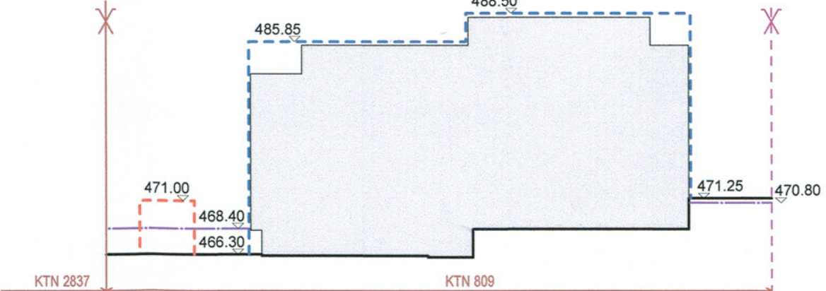
Schnitt B-B
