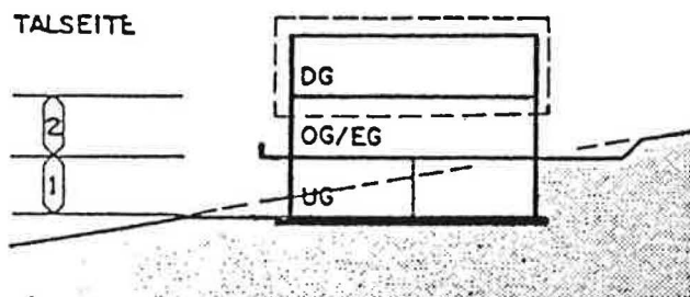
BEISPIEL 1: STELLUNG MIT GIEBELSEITE GEGEN DAS TAL
