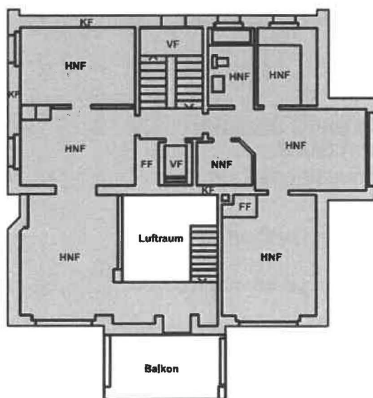
Abbildung Geschossflächen
